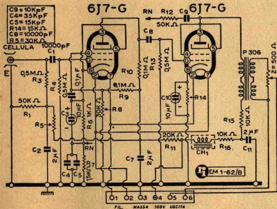
Preamplificatore per "AC 3000,, e "D 65 PN,,
